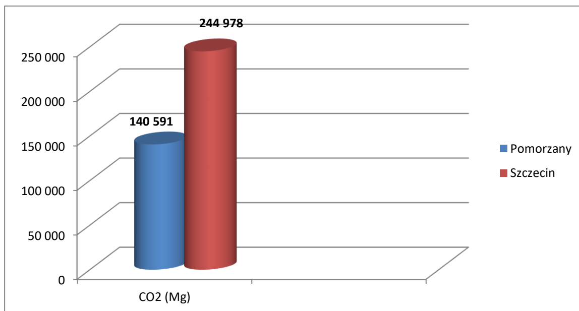
Rysunek 2 Emisje dwutlenku węgla w poszczególnych elektrociepłowniach
