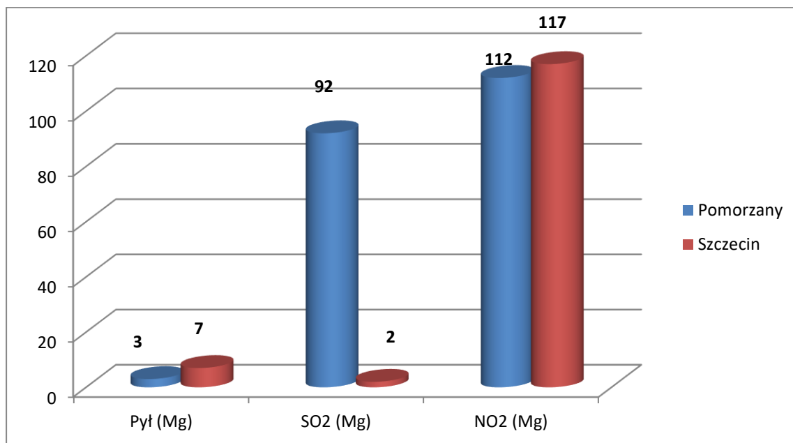
Rysunek 1 Emisje pyłu, dwutlenku siarki oraz tlenu azotu w poszczególnych elektrociepłowniach
