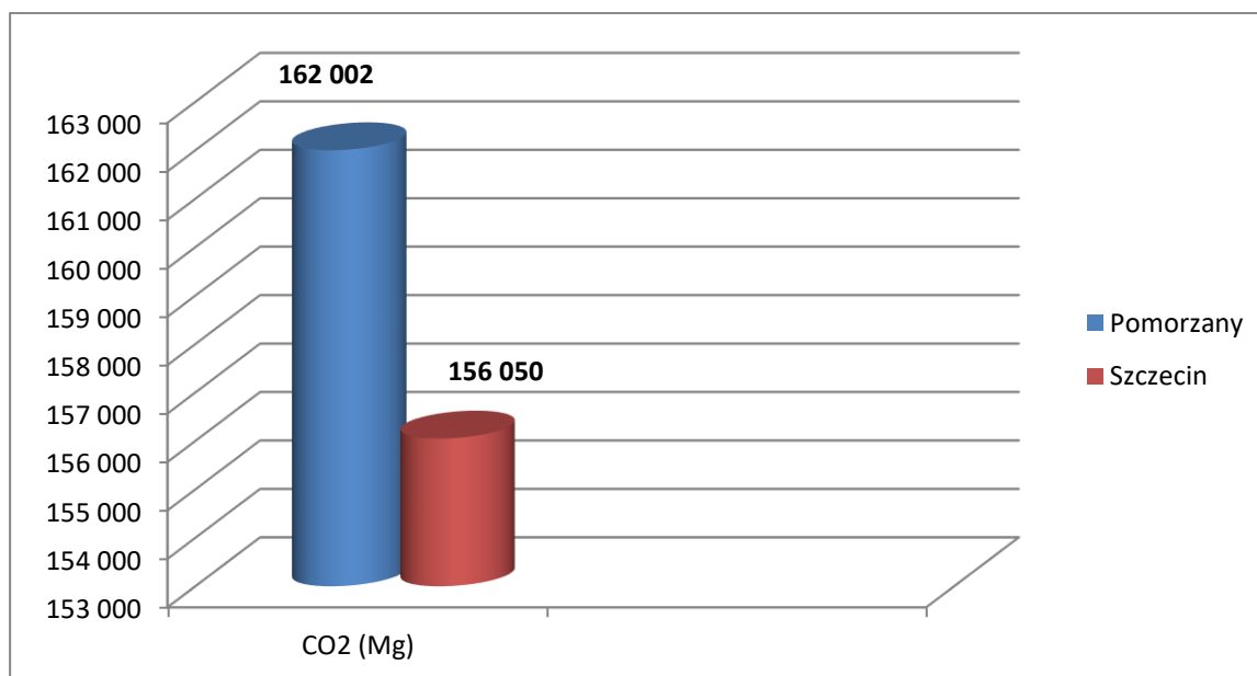
Rysunek 2 Emisje dwutlenku węgla w poszczególnych elektrociepłowniach
