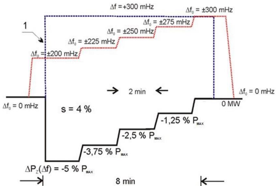
Rys. 4 Sprawdzenie odpowiedzi częstotliwościowej przy zmianach: strefy nieczułości odpowiedź częstotliwościowej, statyzmu oraz odchyłki częstotliwości.
